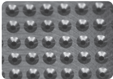
微細穴加工例
